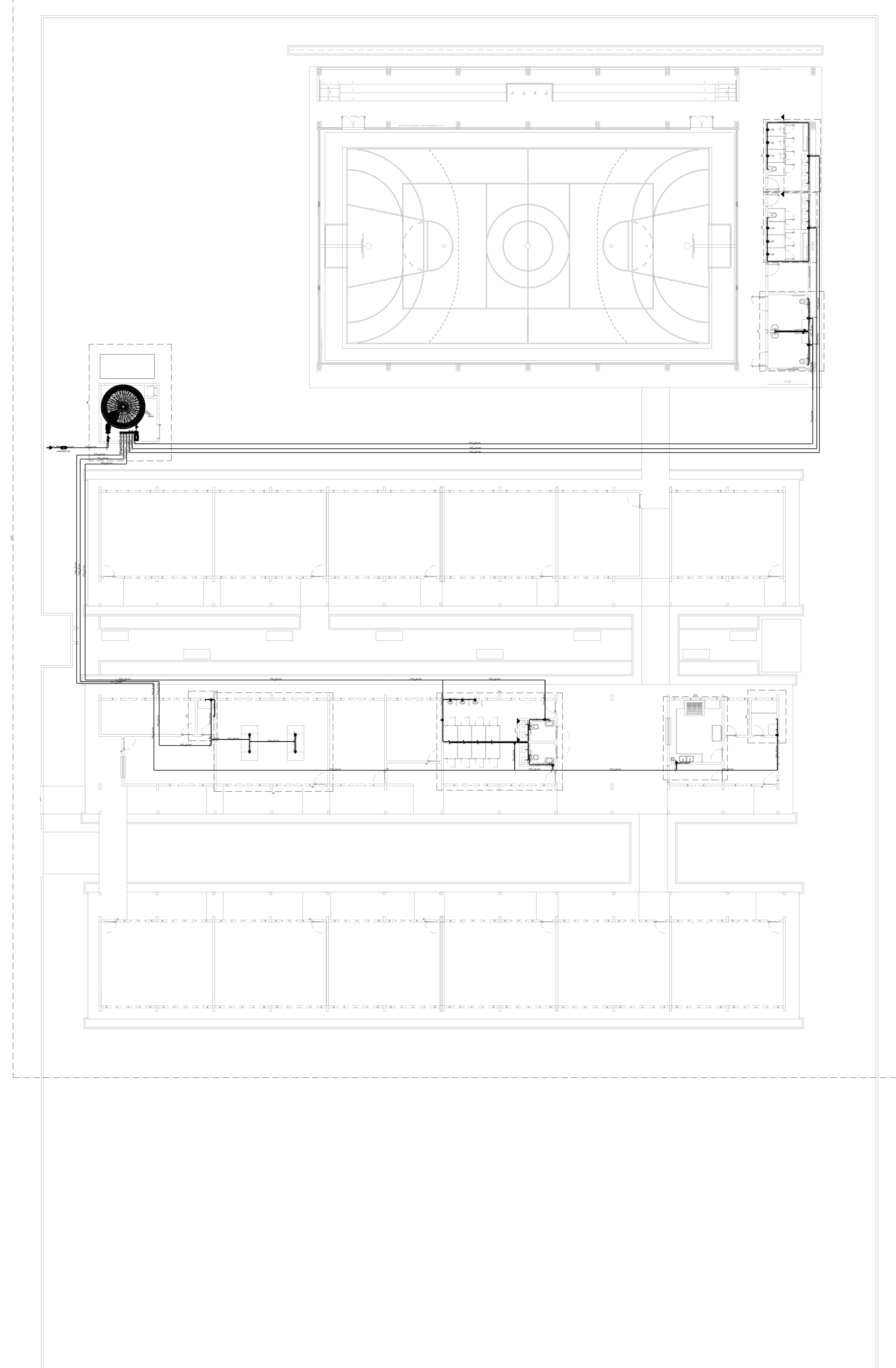
PLANTA BAIXA DE DETALHES HIDRÁULICO
