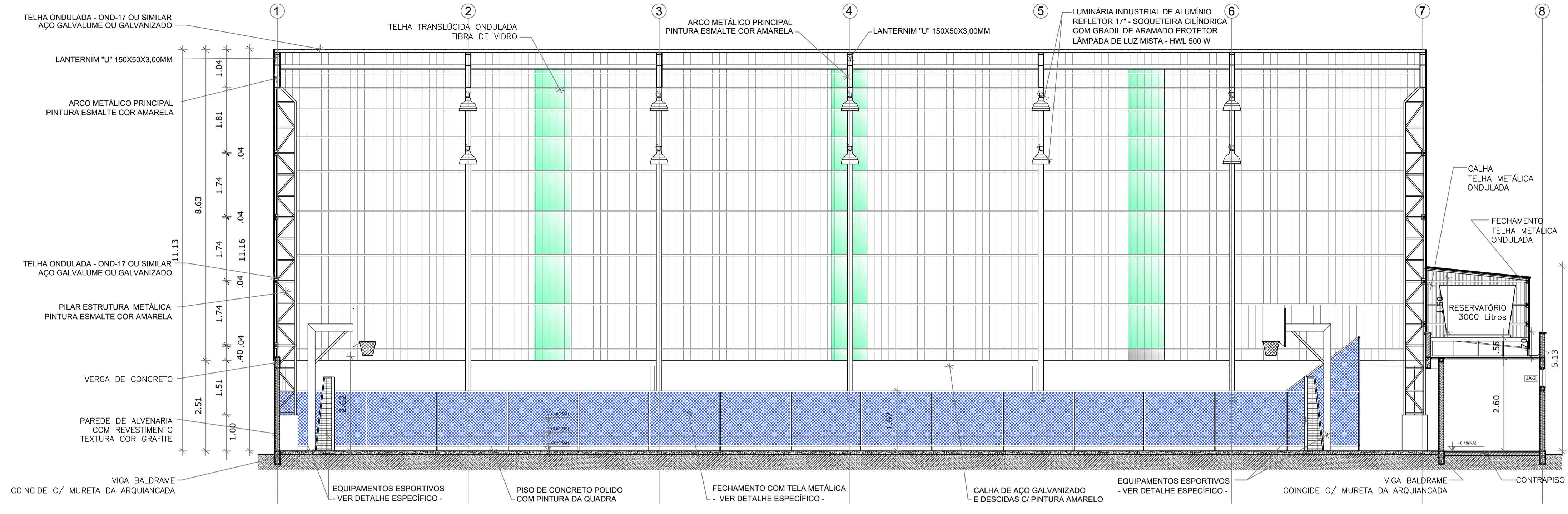
1 CORTE AA' ESCALA 1/75
