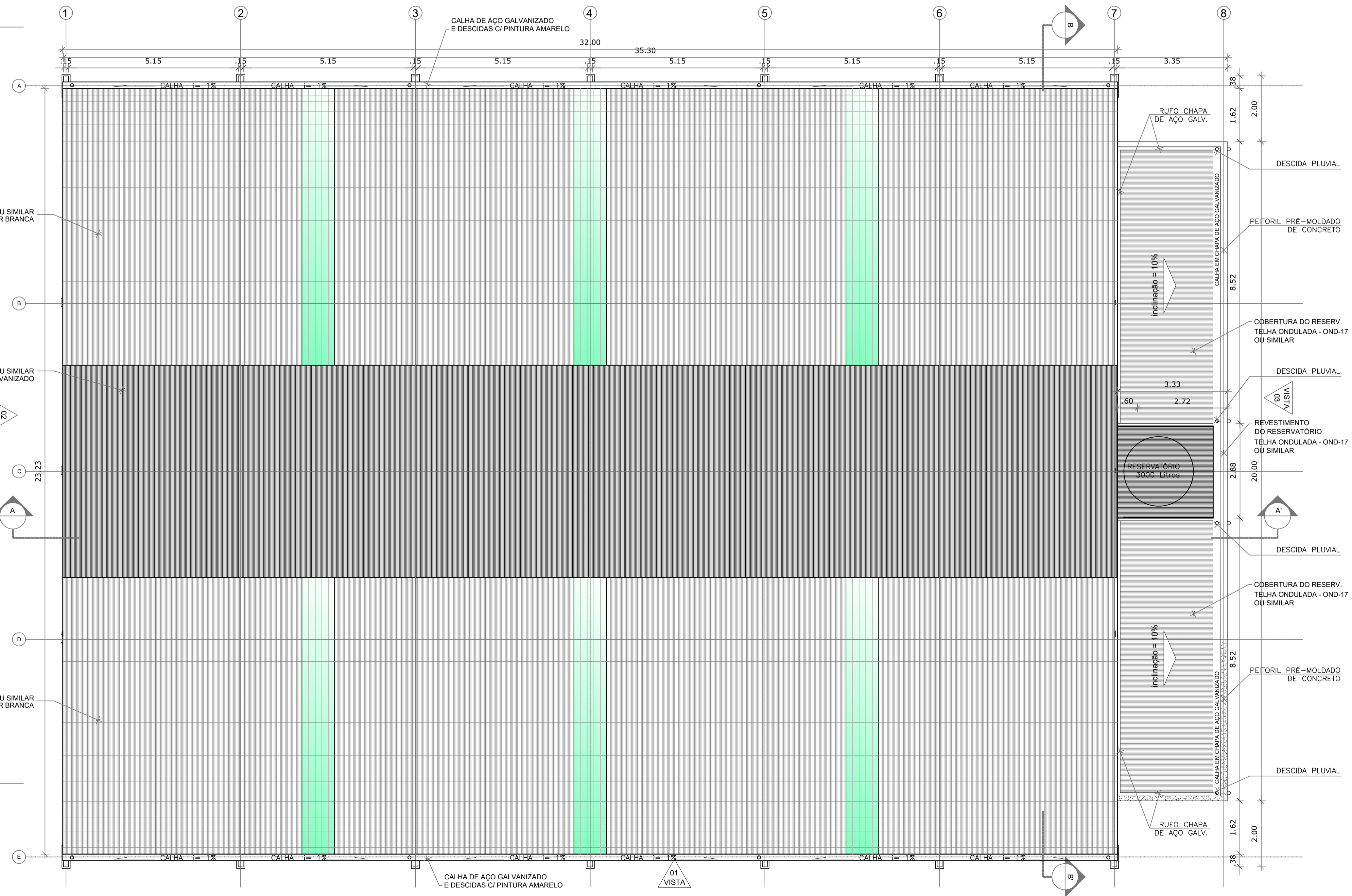
2 COBERTURA ESCALA 1/75
