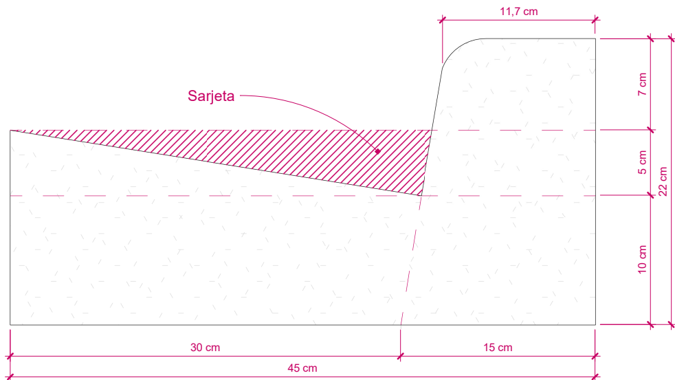
1 Detalhamento da Sarjeta e Meio-fio Conjugados ESCALA: 1 : 4
