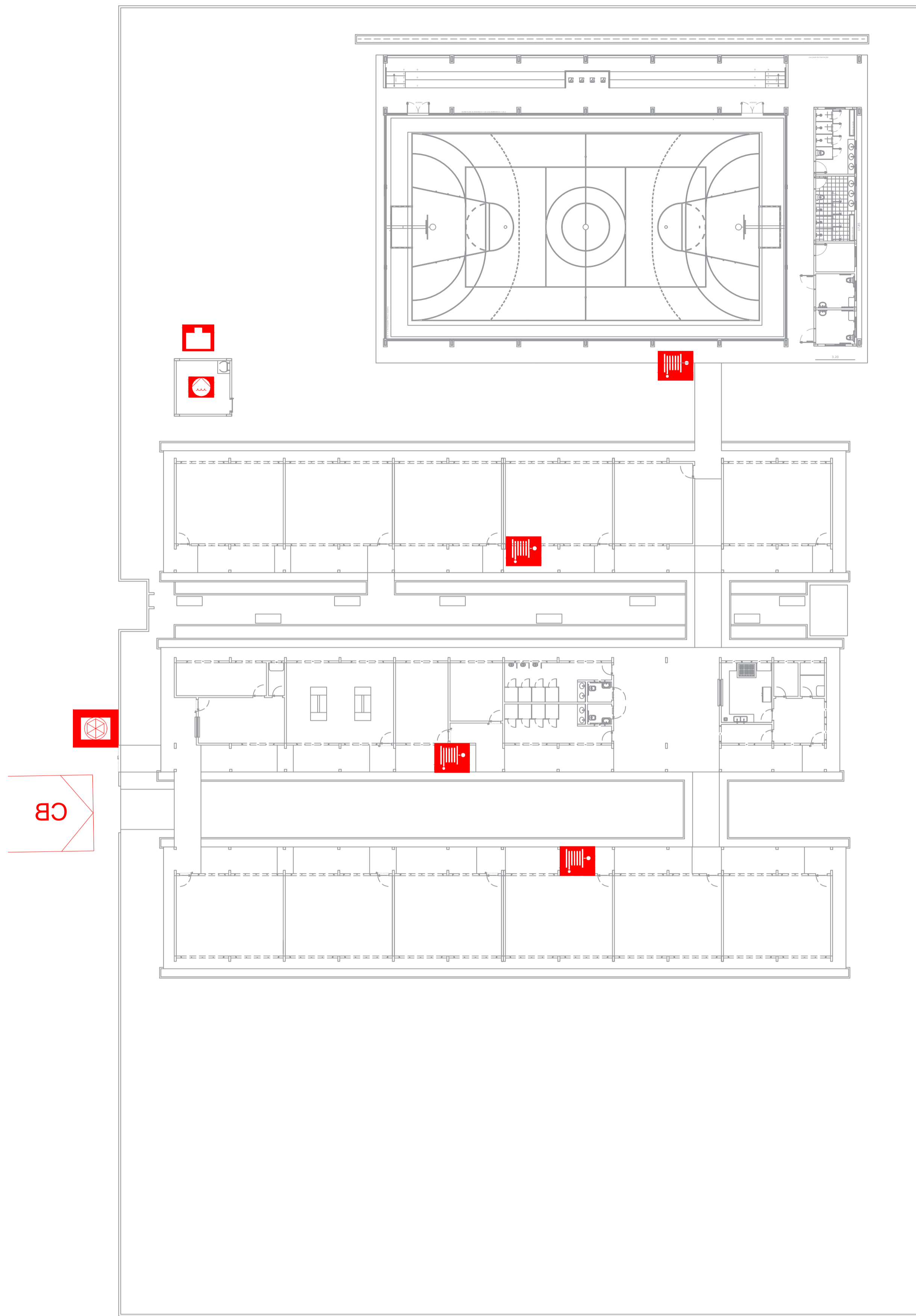
PLANTA DE RISCO escala.....1:150
