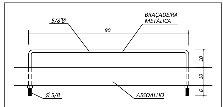
Detalhe 03
