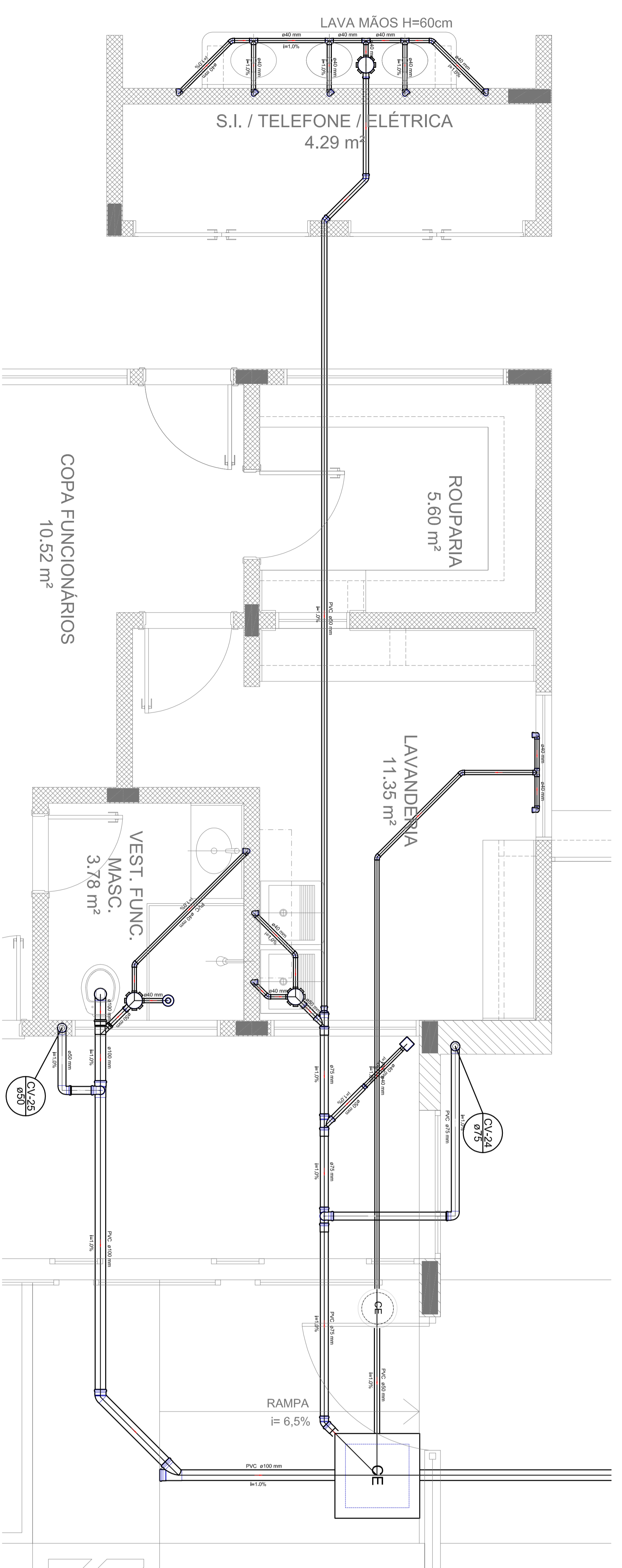
Detalhe S15 escala 1:25
