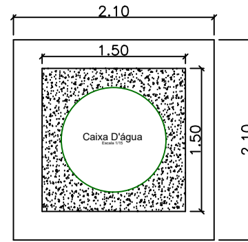
Planta Baixa Escala 1/10
