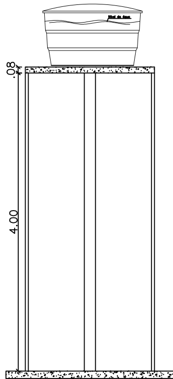
Det. Esquema Cx D'água Escala 1/10
