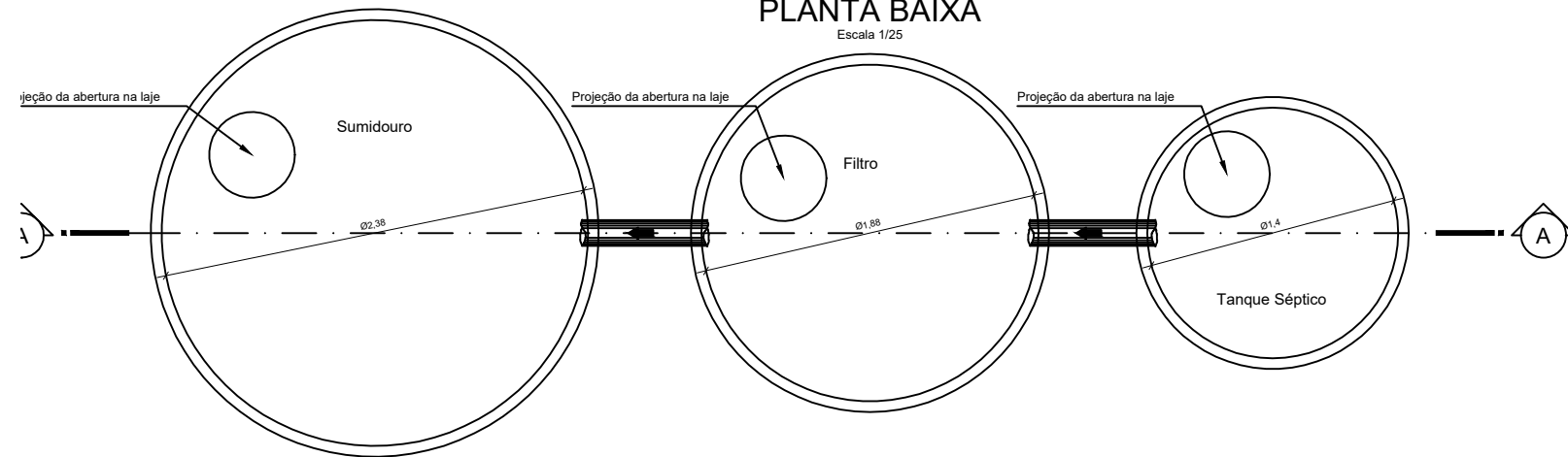
DET. 01 - SISTEMA FOSSA/FILTRO/SUMIDOURO PLANTA BAIXA
