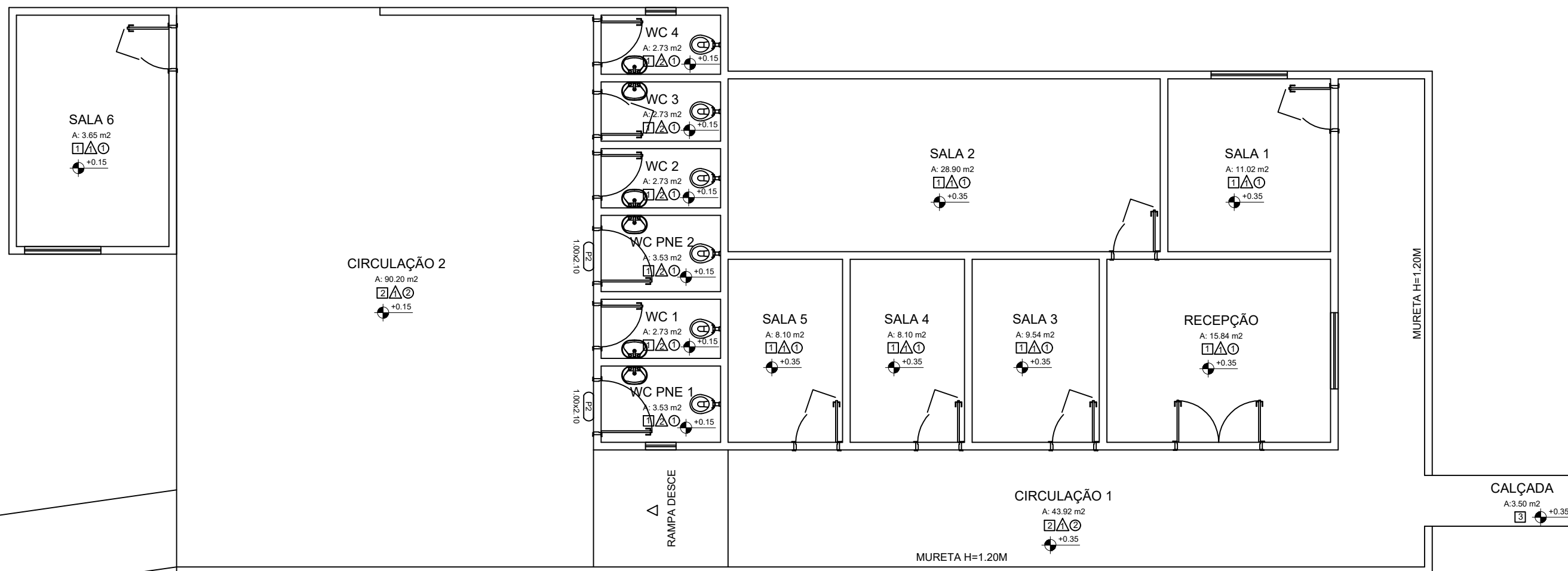
PLANTA BAIXA EXISTENTE (PRÉDIO) Escala 1/75
