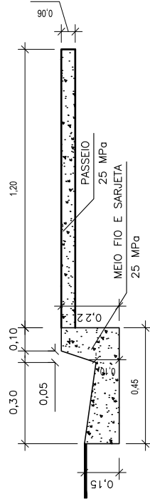
DETALHE PADRÃO DETALHE DE SARJETÃO ESC. = 1/10
