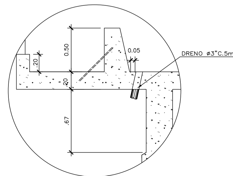
DETALHE C ESCALA: 1/25
