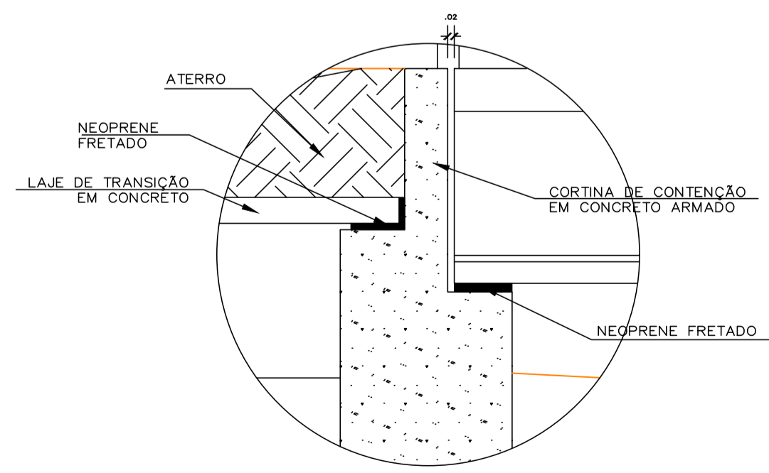
DETALHE A ESCALA: 1/25
