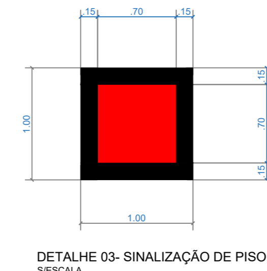
DETALHE 03 - SINALIZAÇÃO DE PISO ESCALA
