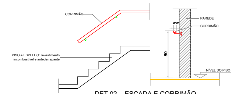
DET.02 - ESCADA E CORRIMÃO ESCALA
