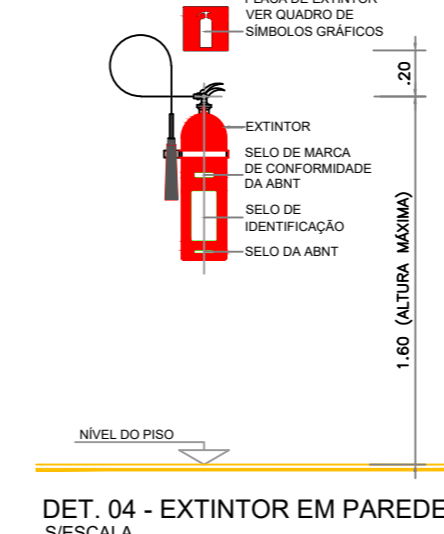
DET.04 - EXTINTOR EM PAREDE ESCALA
