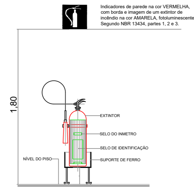
DET.01 - EXTINTOR SOBRE BASE ESCALA
