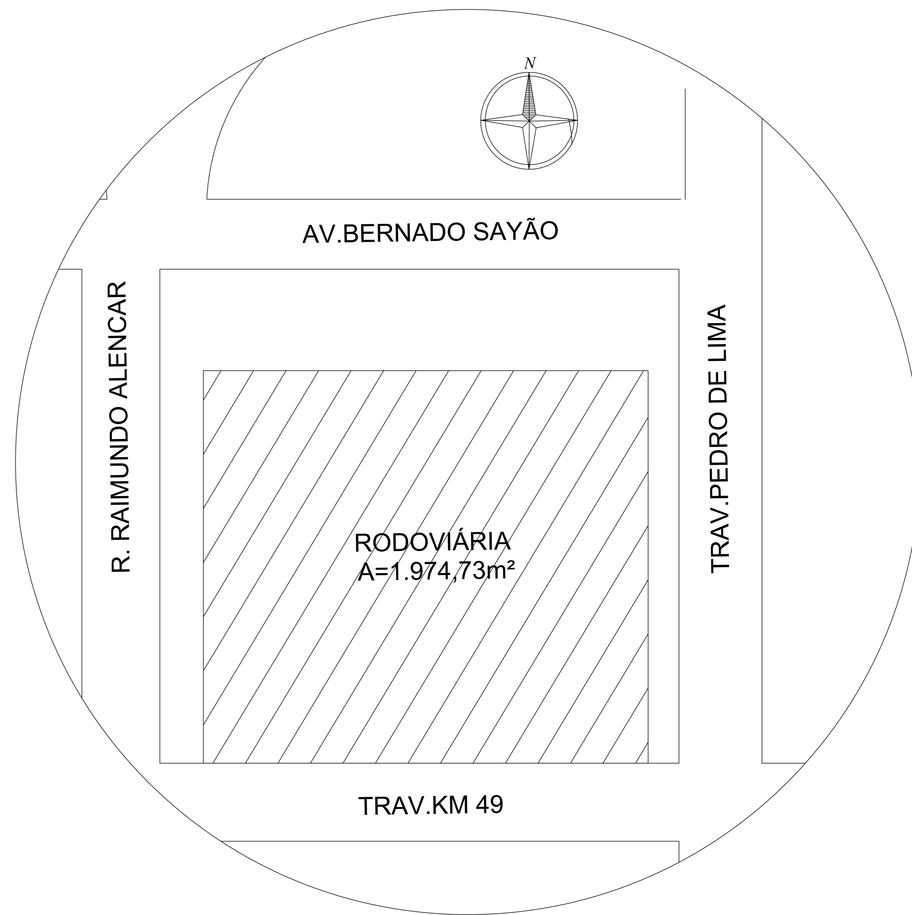
PLANTA DE SITUAÇÃO E LOCAÇÃO - S/ESC.
