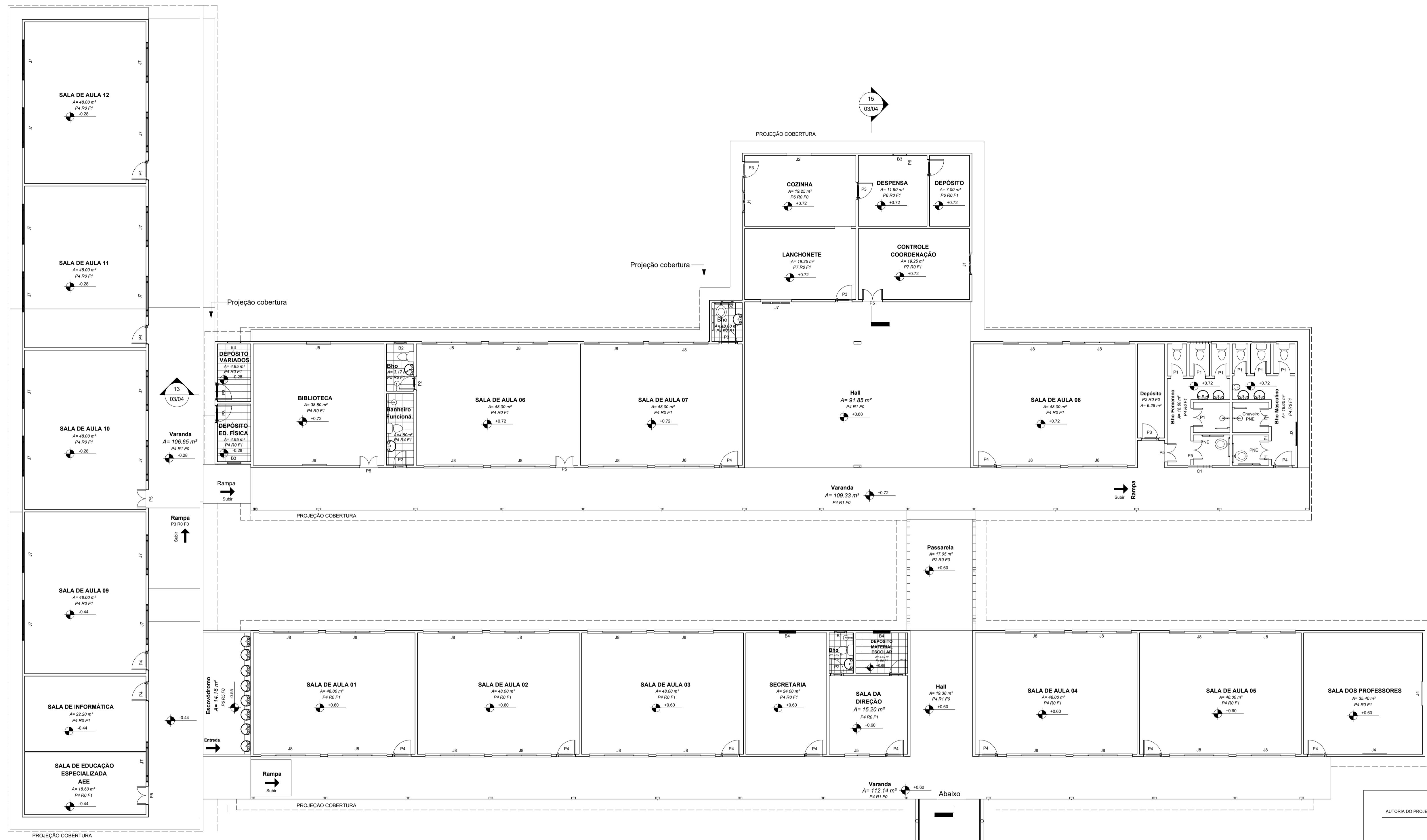
PLANTA DE BAIXA ATUAL- ESC. 1:100
