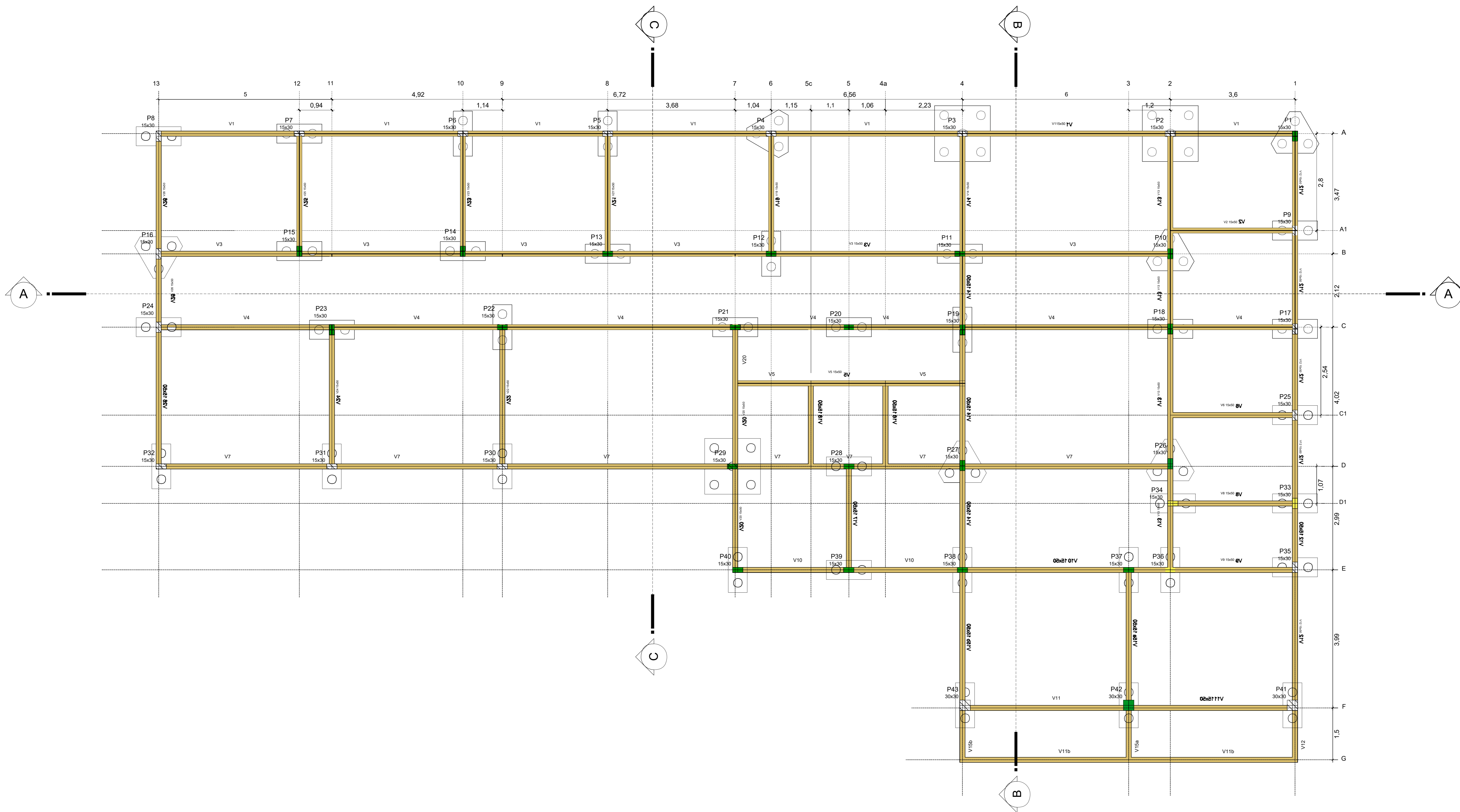
LOCAÇÃO VIGAS BALDRAMES Escala: 1/75
