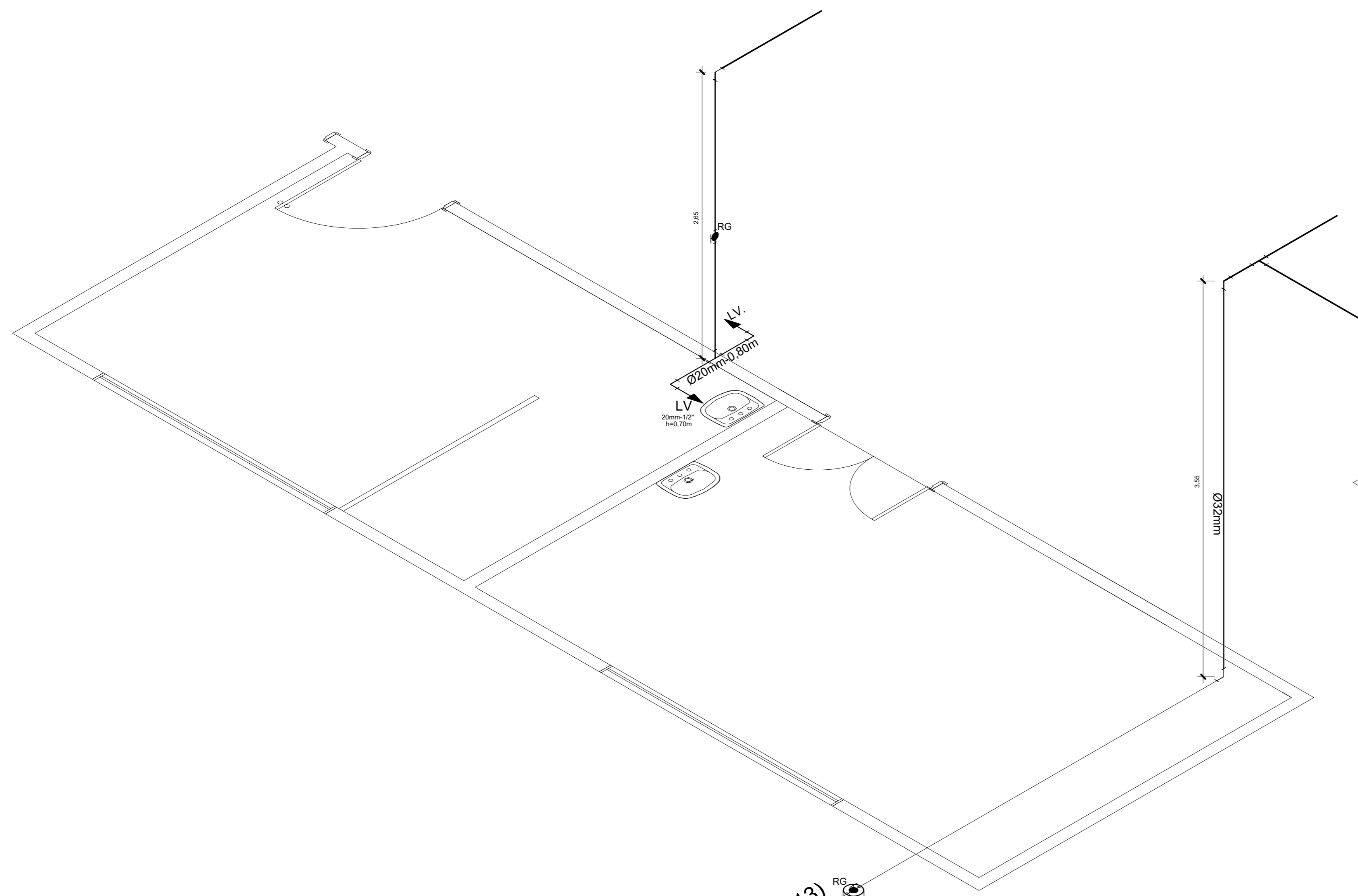
Isometria - Sala Ex.Indif Isometria - Sala de Reidratação Escala 1/25
