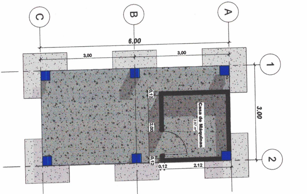
② 01 - Térreo 1:75
