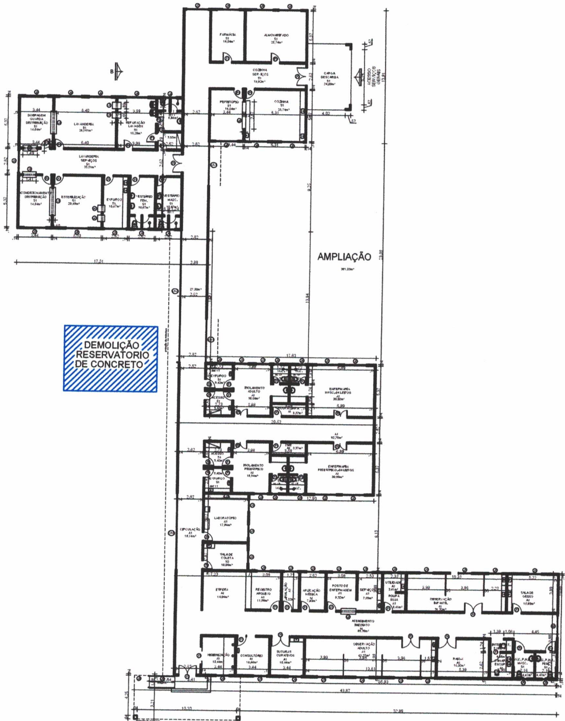
PLANTA BAIXA TÉCNICA ESCALA: sem escala
